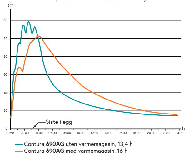
Temperaturkurver Contura 690AG Style
