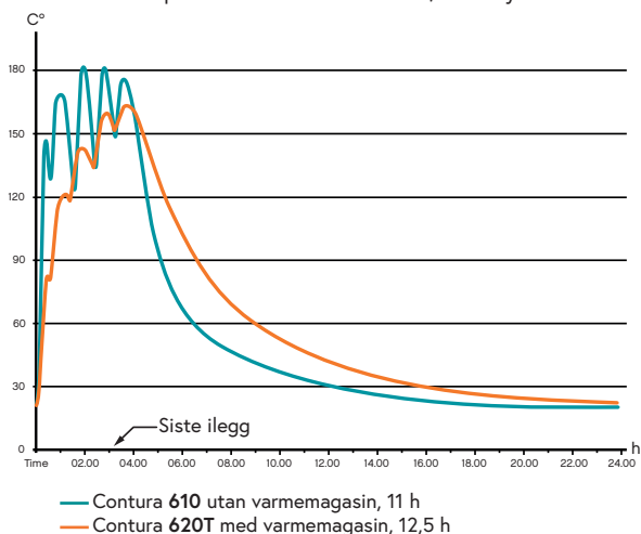
Temperaturkurver Contura 620T / 610 Style
