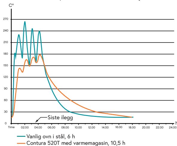
Temperaturkurver Contura 520T Style
