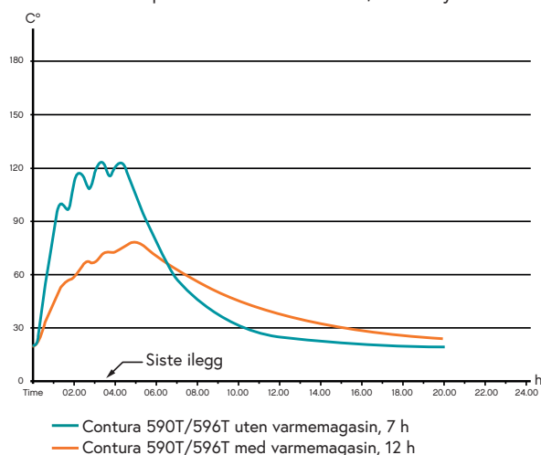
Temperaturkurver Contura 590 / 596T Style
