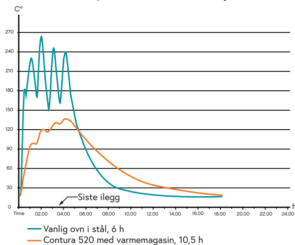
Temperaturkurver Contura 520 Style
