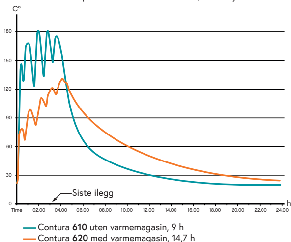
Temperaturkurver Contura 620 / 610 Style
