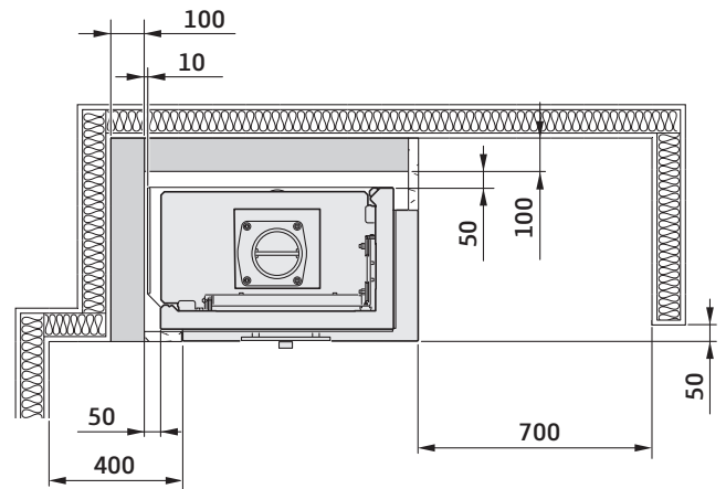
Parete in materiale ignifugo, nell'esempio di rivestimento la parete è in calcestruzzo aerato da 100 mm.
