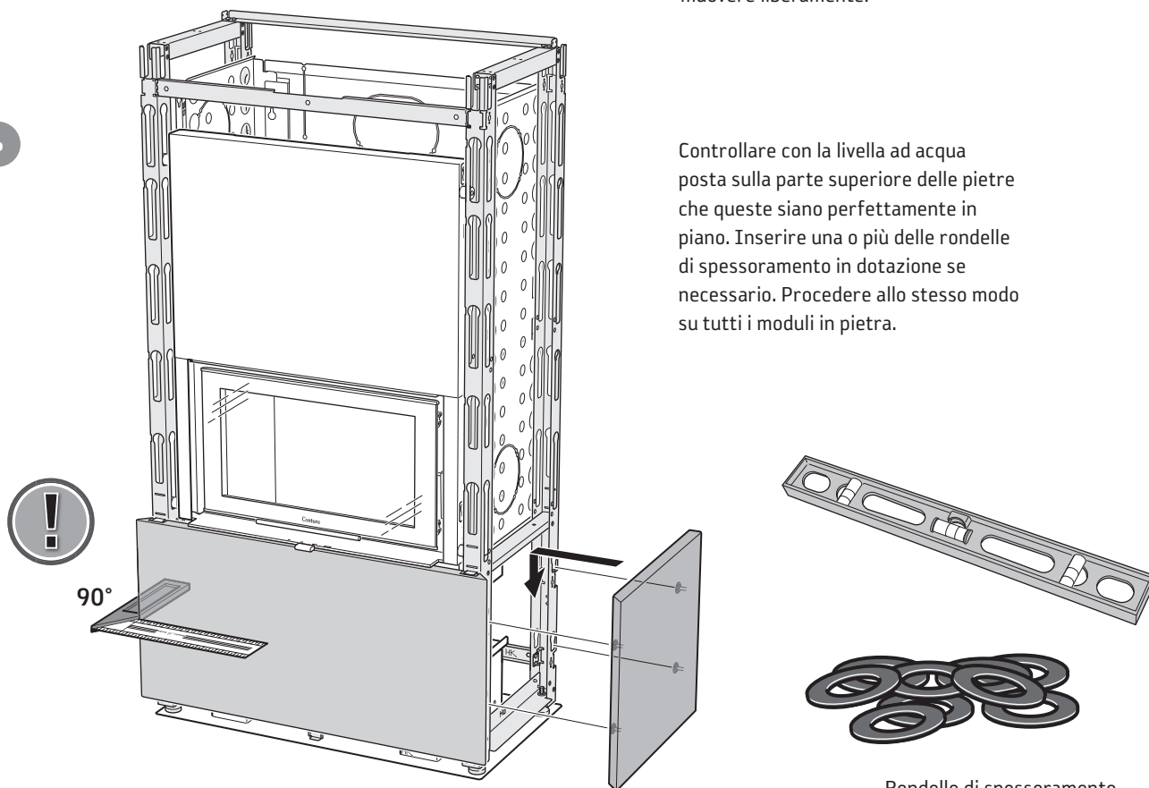
Rondelle di spessoramento
