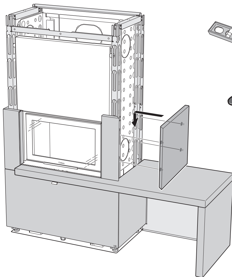
Rondelle di spessoramento
