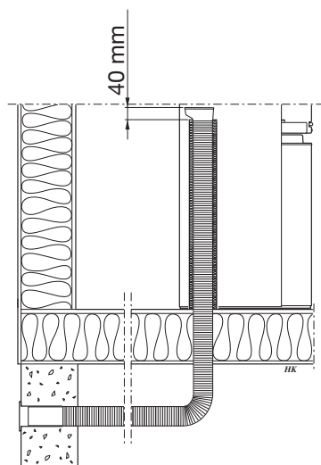
Via gulv og krybekælder
