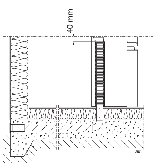
Via gulv og fundament
