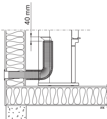
Gjennom yttervegg.
