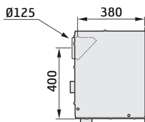
Tilkoblingsmål
