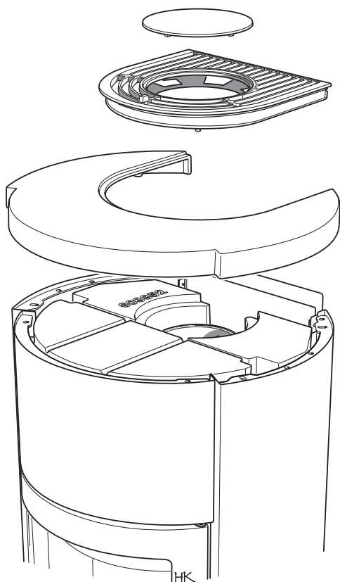
Avec accumulateur de chaleur. Monter la grille de diffusion d'air chaud réglable.
