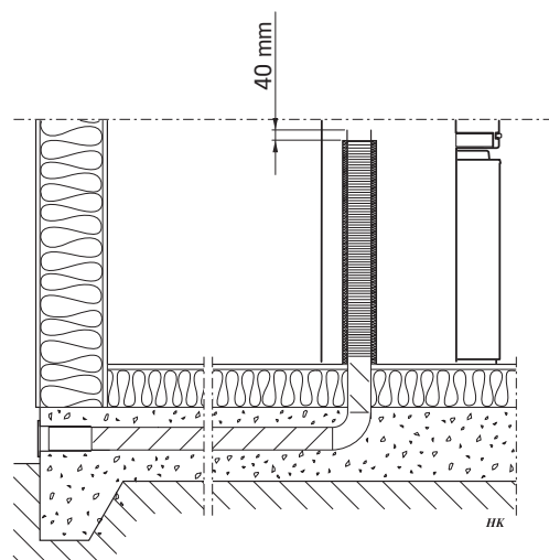
À travers le plancher et la dalle en béton.
