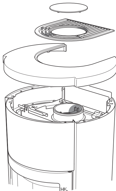
Sans accumulateur de chaleur. Monter la grille de diffusion d'air chaud standard.
