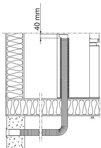
À travers le plancher et le vide sanitaire
