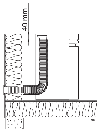
À travers le mur extérieur
