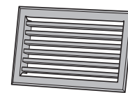
Varmluftsgaller inbyggnadsmått 255x130 mm, genomsläppsarea 150 cm 2
